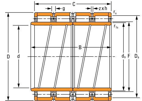
RX-6
