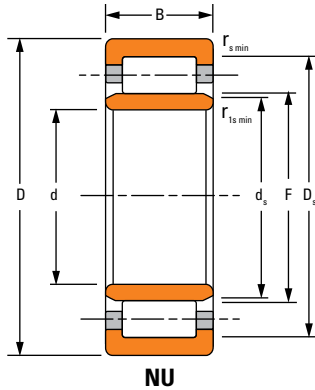
NU
