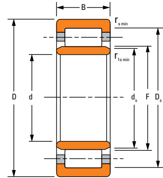
NU
