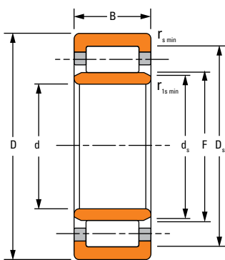
NU
