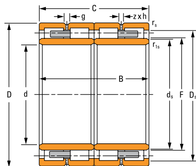
RY-2, RYL-2
