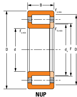
NUP
