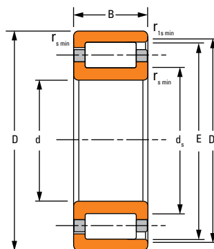
NF
