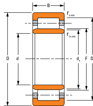
NU
