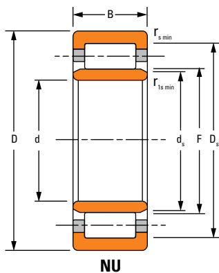
NU
