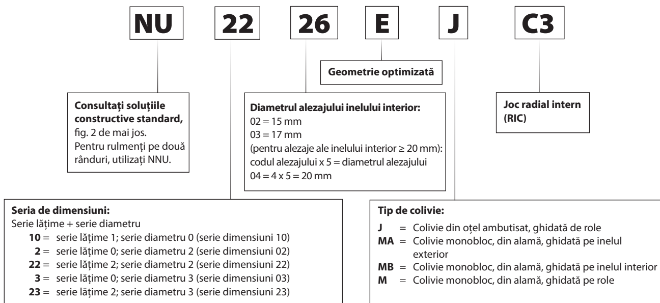
Fig. 1. Simbolizarea în sistem metric ISO pentru rulmenții radiali cu role cilindrice.
