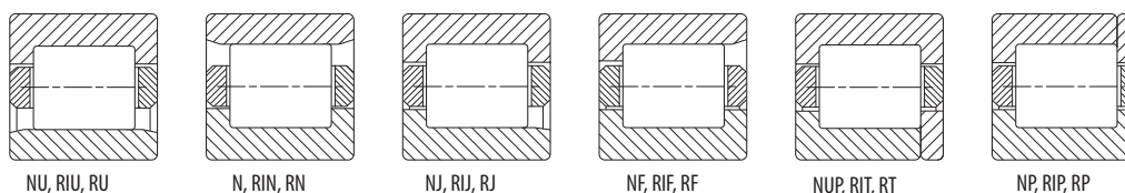
Fig. 2. Soluții constructive de rulmenți radiali cu role cilindrice standard în sistem metric/imperial.
