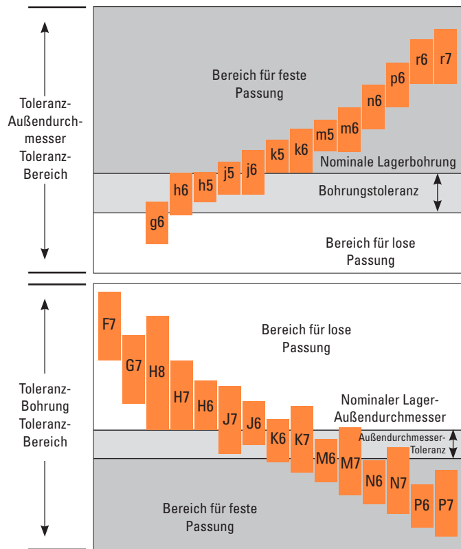
Abb. 5. Passungsauswahl für Welle und Gehäuse.
