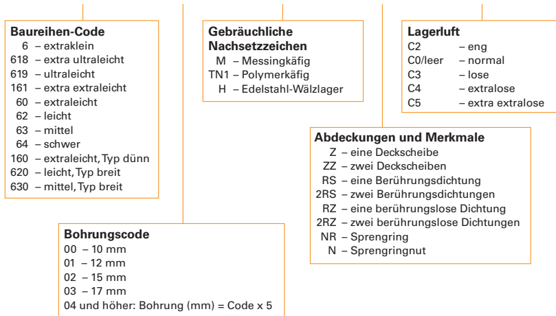
Abb. 1. Bezeichnungssystem für Rillenkugellager
