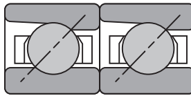
Tandem DT
