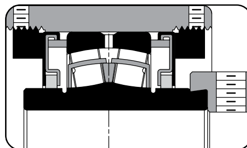
Fig. 14. T seal.
