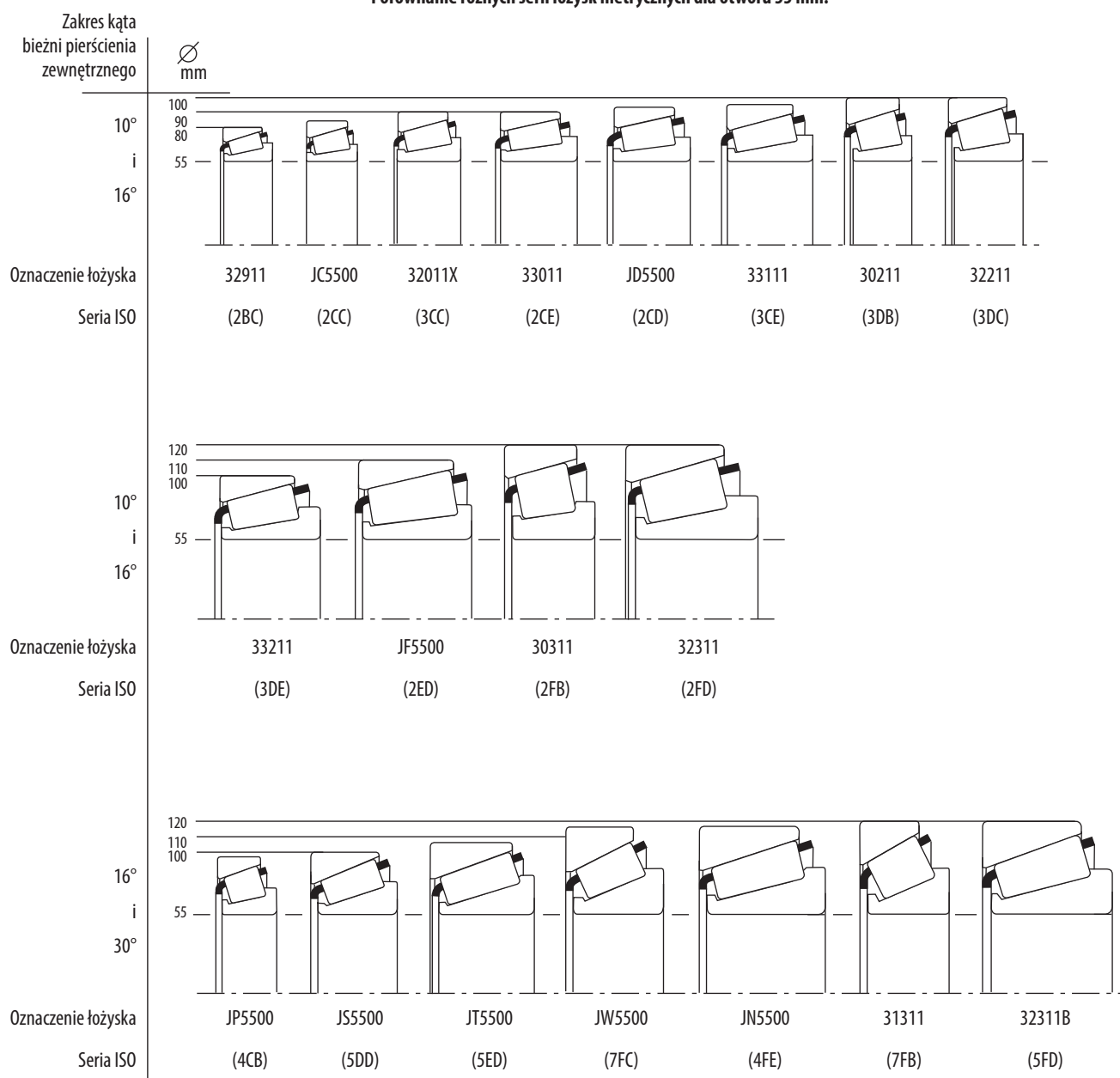
Porównanie różnych serii łożysk metrycznych dla otworu 55 mm.
