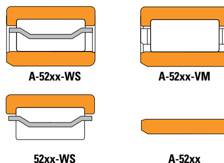
Abb. 2. Lager der metrischen Baureihe 5200
