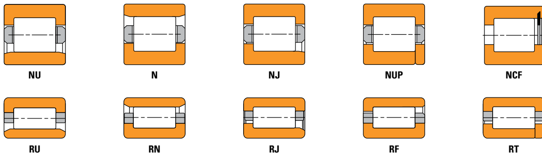
Abb. 18. Bauarten metrischer/zölliger Standard-Zylinderrollenlager
