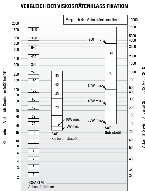
Abb. 13. Vergleich zwischen ISO/ASTM-Klassen (ISO 3448/ASTM D2442) und SAE-Klassen (SAE J 300--80 für Kurbelgehäuseöle, SAE J 306--81 für Achs- und Schaltgetriebeöle).
