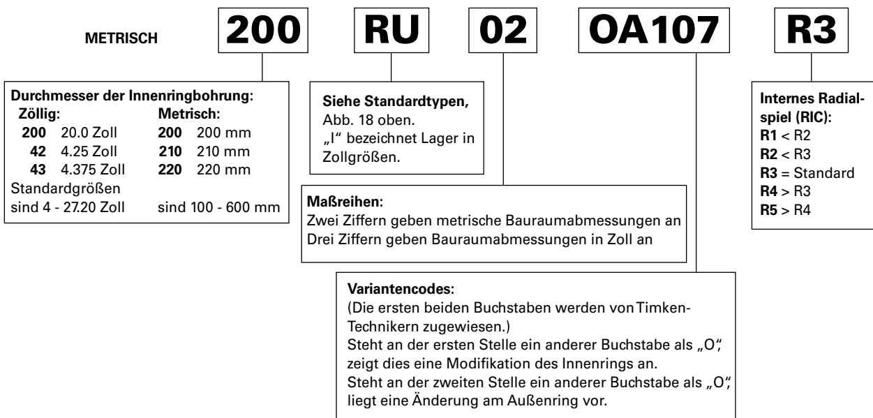
Abb. 19. Bezeichnungen Radialzylinderrollenlager nach ABMA.
