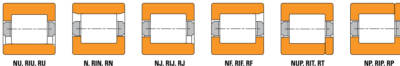
Abb. 1. Radial-Zylinderrollenlager.
