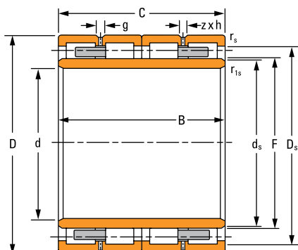
Abb. 23. Zylinderrollenlager.
