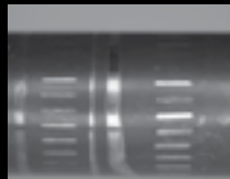
Falso brinelling di un albero sul quale è stato montato un cuscinetto a rulli cilindrici
