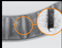
Falso brinelling. Solchi d'usura profonda sulla pista di un anello esterno
