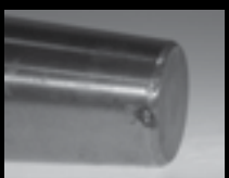
Rullo con bruciature da arco elettrico
