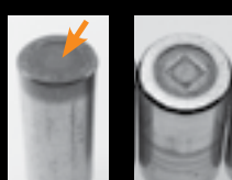
Sovratemperatura sviluppata in corrispondenza della testa sferica dei rulli/bordino dell'anello interno
